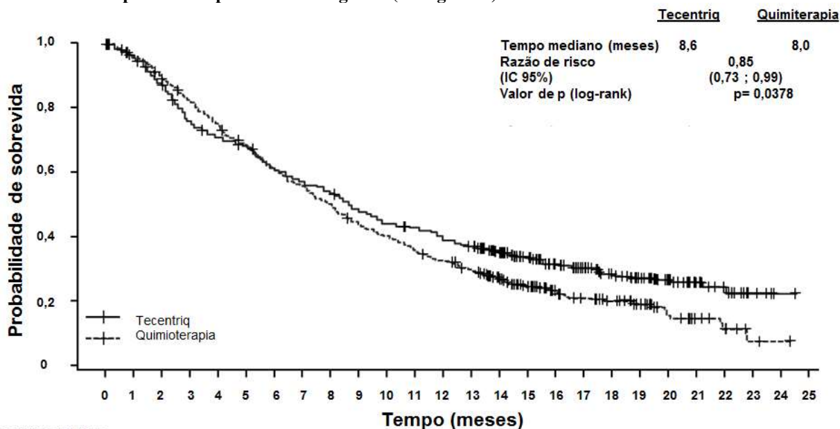
Figura 1: Gráfico Kaplan-Meier para sobrevida global (IMvigor211)
