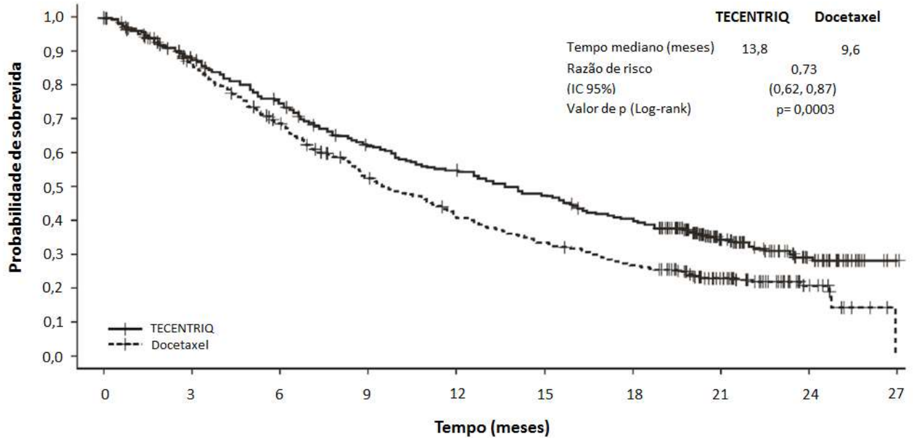
Figura 2 – Gráfico de Kaplan-Meier para sobrevida global na população da análise primária (todos os pacientes, independentemente da expressão de PD-L1) (OAK)
